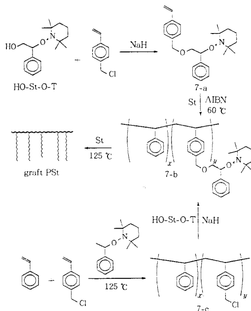
그림 7. Synthesis of graft PSt by 'living' FRP using nitroxide unimolecular initiators.
