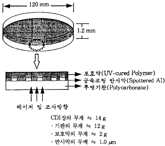
그림 2. 일반 음악용 CD의 구조.
