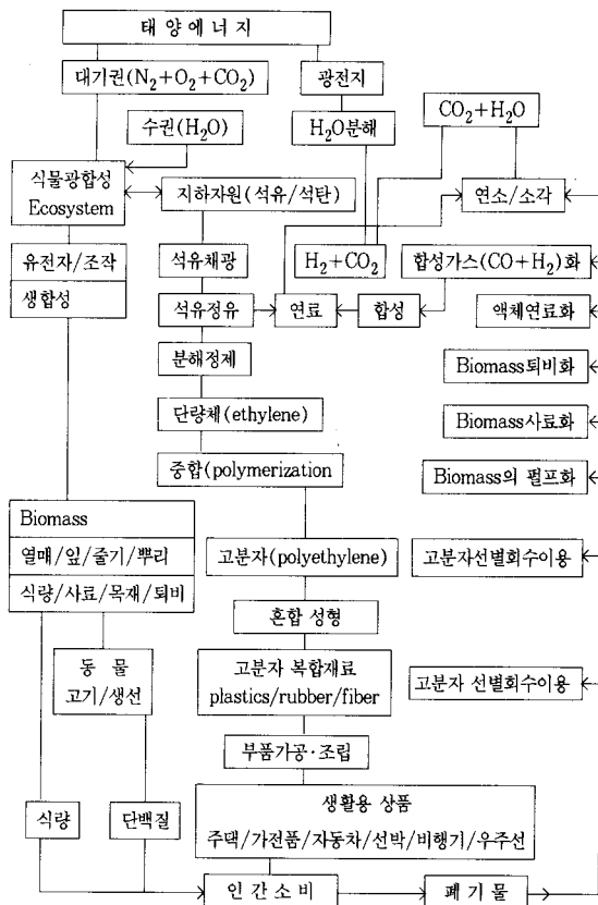
그림 1. 유기제품의 순환 과정과 환경 친화성 평가 모델(life-cycle assessment).
