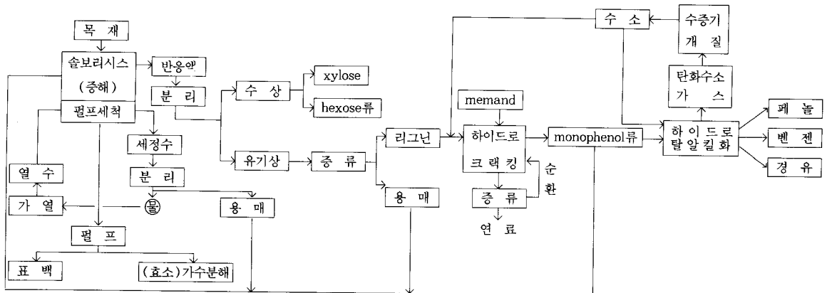
그림 12. 술볼리시스 공정.
