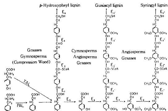
그림 9. Monolignol의 생합성.
