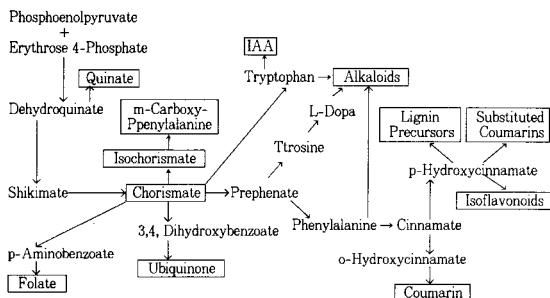
그림 8. Shikimate 경로.
