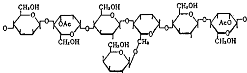
O-acetyl-galactoglucomannan( 침엽수 헤미셀룰로오스의 주제 )
