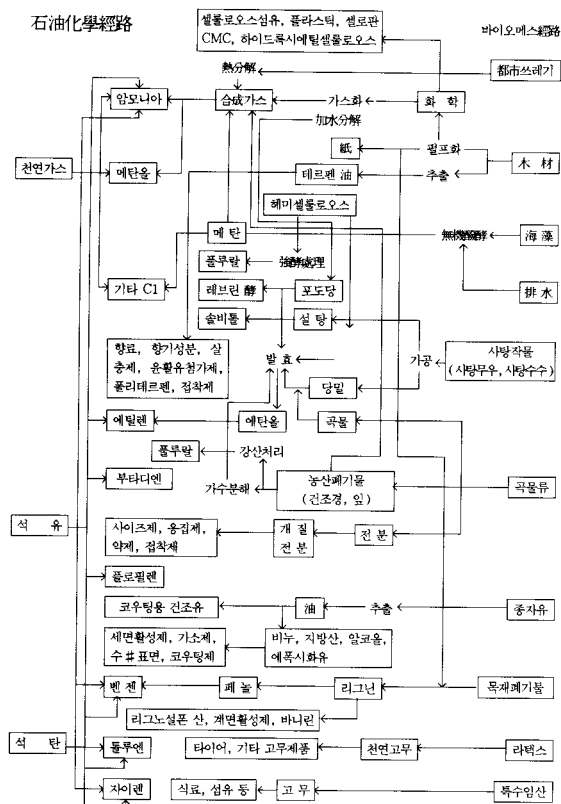
그림 15. 석유화학 및 바이오메스로부터 유기화학제품의 제조경로.
