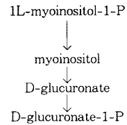
그림 2. Myoinositol 산화경로에 의한 pectin의 합성(Loewus, 1973).
