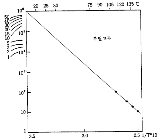
그림 2. 단층 쉬이트의 신장률 변화율(-20%에 이르기까지의 시간과 온도의 관계).
