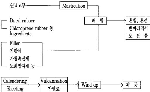
그림 1. 가황제 단층 슈이트의 제조공정 예.
