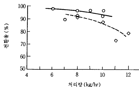
그림 20. Polyoxymethylene의 중합 반응 결과.
