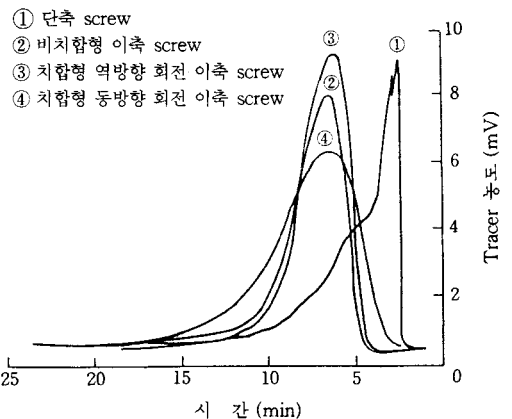
그림 8. 각종 압출기의 체류시간 분포 비교 (동일 screw 형태).
