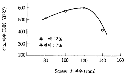
그림 18. Nylon 분자량과 screw 회전수와와의 관계(치합형 이축 screw).
