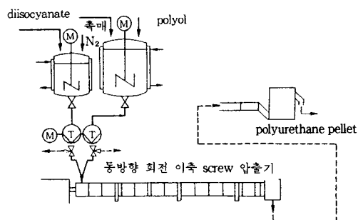
그림 15. Polyurethane의 이축 screw 압출기를 이용한 제조공정.
