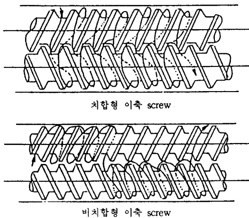
그림 4. Screw 치합에 의한 흐름거동의 차이.
