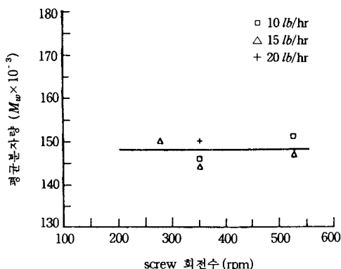
그림 17. Nylon 분자량과 screw 회전수와와의 관계(비치합형 이축 screw).
