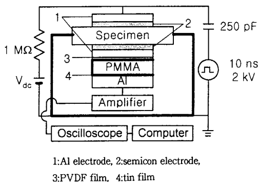
그림 7. Schematic diagram of PEA system.
