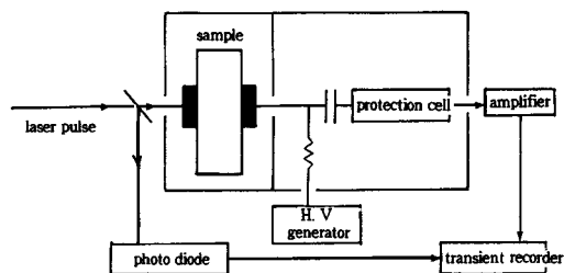
그림 5. Schematic diagram of LIPP method.
