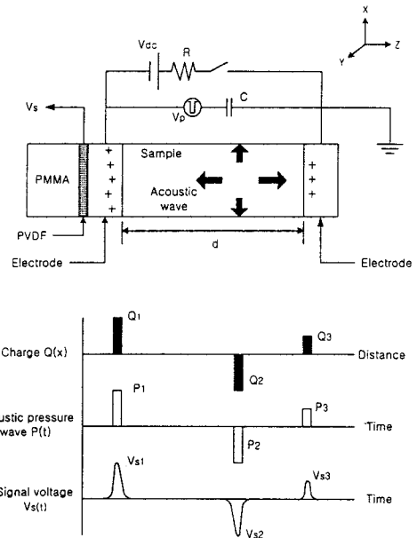
그림 6. The principle of PEA method.
