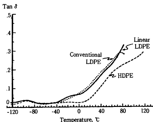
그림 4. Mechanical tan δ of polyethylene. 26
