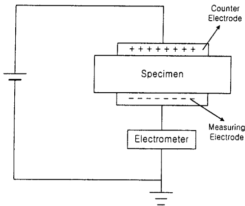
그림 9. Circuit for measuring electrical conductivity.
