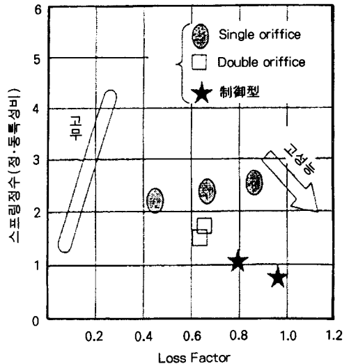
그림 2. 방진고무의 동특성MAP.
