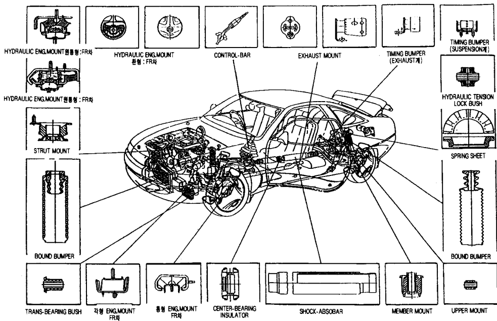
그림 1. 자동차용 방진고무.
