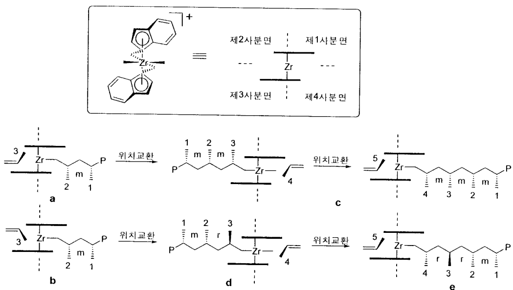
그림 6. rac -(EBI) \text{ZrX}_2 (EBI=1,2-bisindenylethane) 촉매에 의한 프로필렌의 이소타틱성 성장반응기구.
