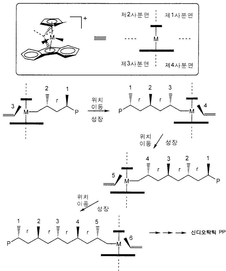
그림 8. i\text{Pr}(\text{Cp})(\text{Flu})\text{MX}_2 ( \text{Flu}=\text{fluorenyl} ) 촉매에 의한 프로필렌의 신디오택틱성 성장반응기구.
