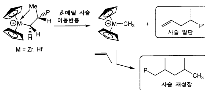
β-메틸 제거반응의 예
