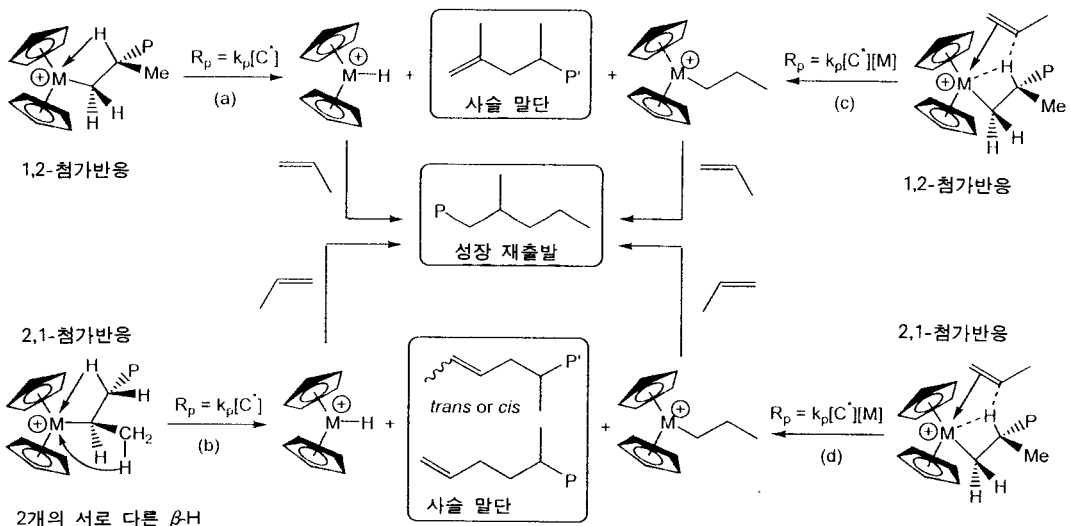
그림 9. 메탈로센 촉매에 의한 프로필렌의 중합에서 흔히 일어나는 성장사슬 전이반응.
