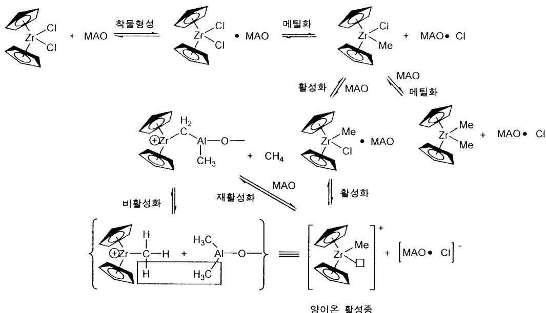
그림 4. 메탈로센/MAO 촉매계의 양이온 활성종 형성기구.
