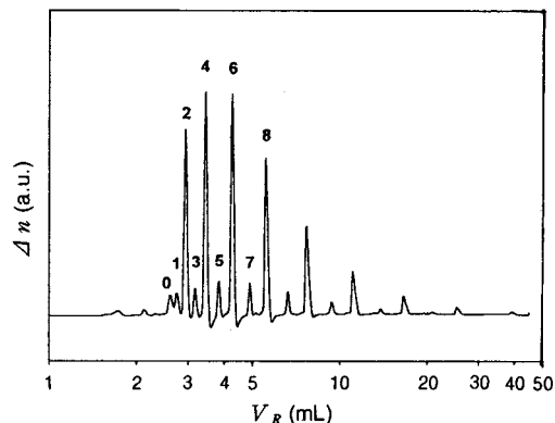
그림 14. PEO임계조건하에 얻은 PEO-PLLA 블록 공중합체의 크로마토그램(봉우리 위에 나타난 번호는 MALDI 질량분석법으로 확인한 PLLA 블록의 중합도를 의미함).
