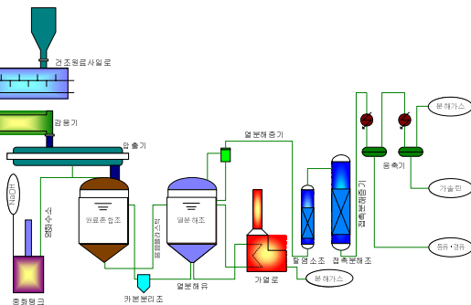
그림 4. 일본 후지리사이클사의 공정도. 6)
