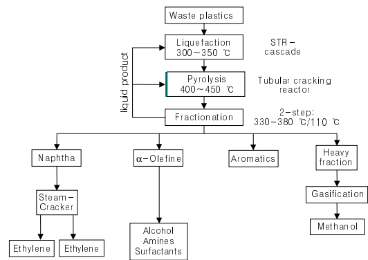
그림 5. 독일 BASF 공정의 Block Diagram. 11
