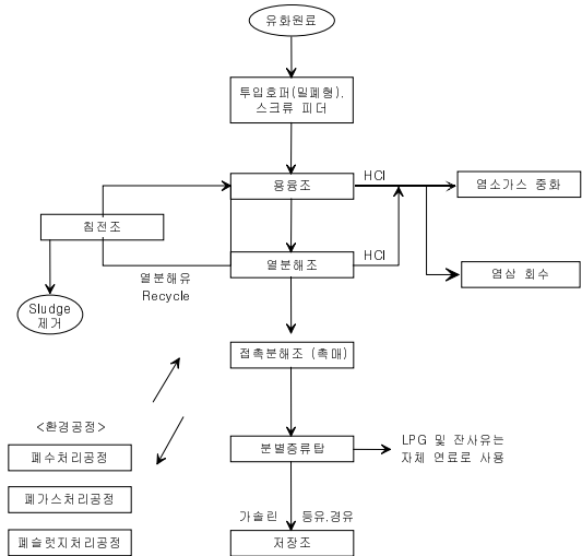
그림 3. 페플라스틱 유화공정의 개념도.
