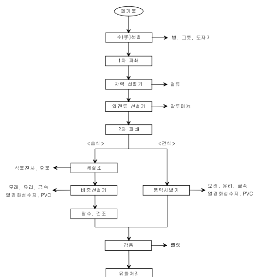
그림 2. 페플라스틱 유화를 위한 전처리 공정 구성 개념도.
