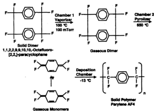
그림 12. Synthesis of parylene AF4 by CVD technique.
