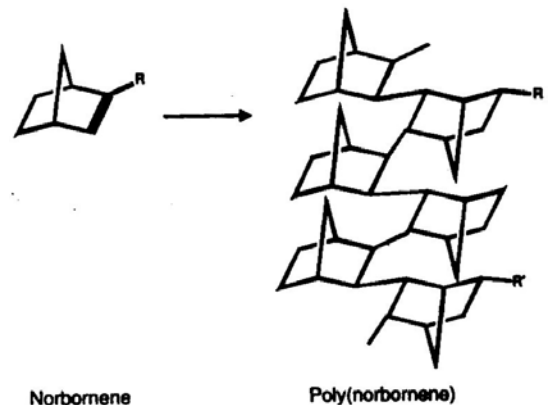
그림 9. Poly(norbornene) derived from cyclic olefine norbornene.
