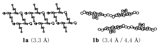
그림 2. 색소 1의 결정 구조 및 층간 거리.
