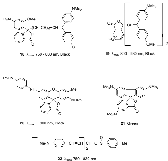
그림 10. 근적외 흡수 색소 전구체.
