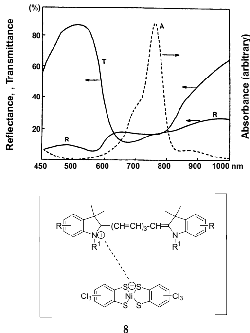
그림 6. Cyanine 색소 8의 흡수 및 반사 특성.
