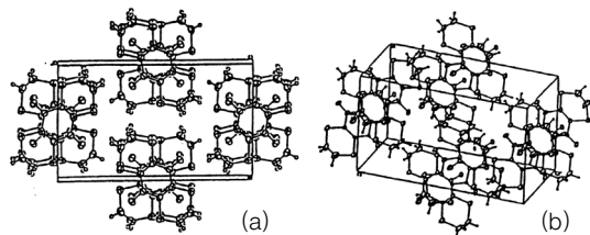
그림 3. 색소 2a의 결정 구조.
