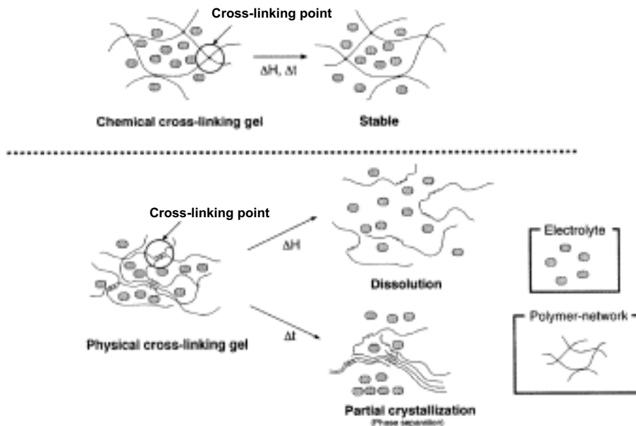
그림 4. Gel-type polymer electrolyte models.
