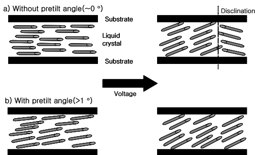
그림 6. 선경사각과 액정 도메인 형성과의 관계.
