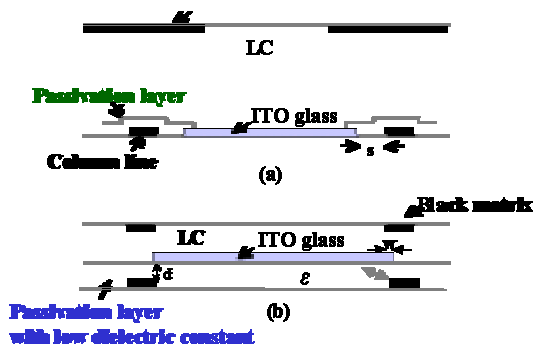
그림 8. 고개구율 LCD의 구조. (a) 기존 LCD device, (b) 고개구율 LCD device.
