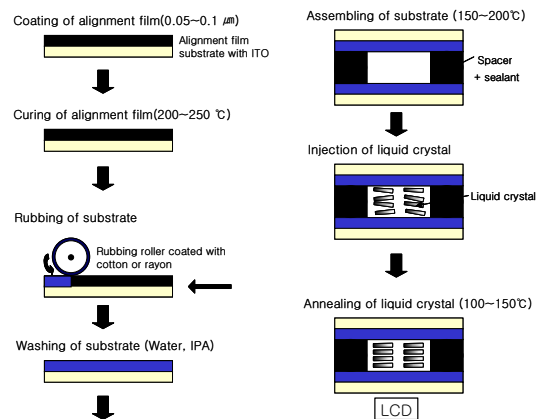
그림 5. LCD의 제작 공정.
