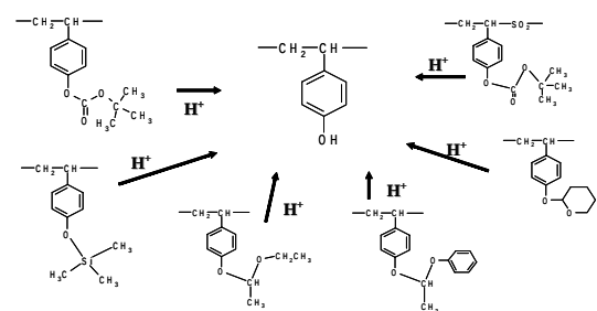
그림 6. KrF 엑시머 레이저(248 nm) 포토레지스트의 보호기.
