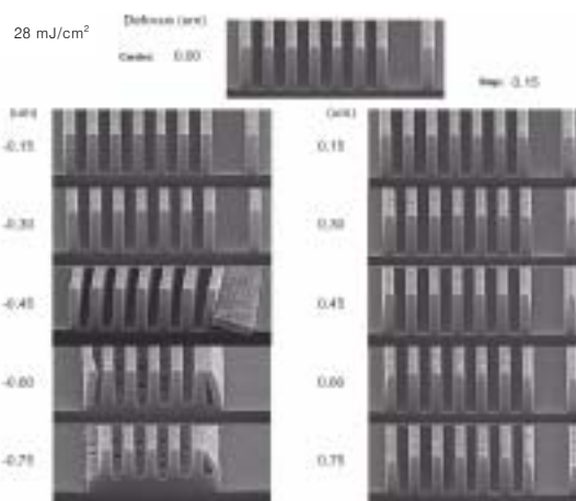
그림 7. 0.2 μm 1:1 L/S DOF margin 단면사진.
