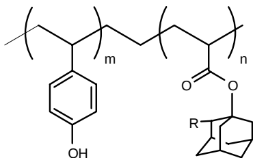
그림 12. EUV 포토레지스트 고분자의 예.
