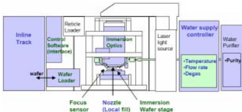
그림 9. ArF immersion 노광시스템(Nikon).
