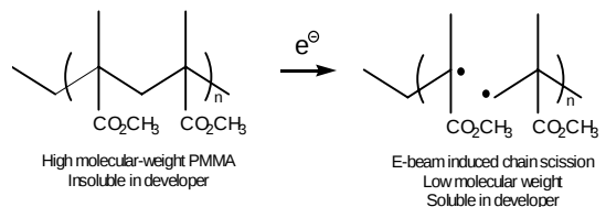
그림 13. 전자 빔을 이용한 PMMA 주사슬 절단 기작. 23
