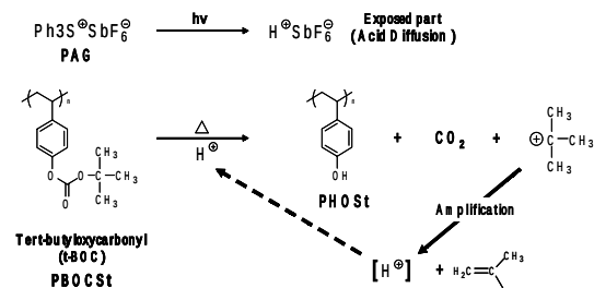
그림 5. KrF 엑시머 레이저(248 nm) 포토레지스트의 작용 기작.
