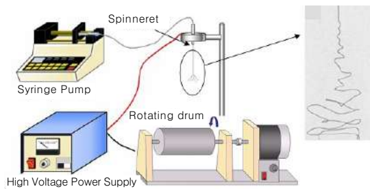
그림 1. 전기방사 장치 및 고분자 jet. 5
