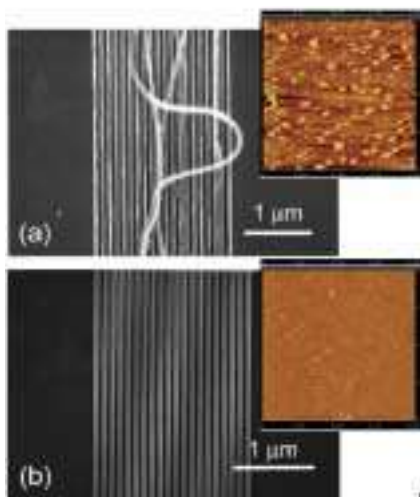
그림 13. 나노임프린트 공정에서 (a)액상법과 (b)기상법의 비교. 18
