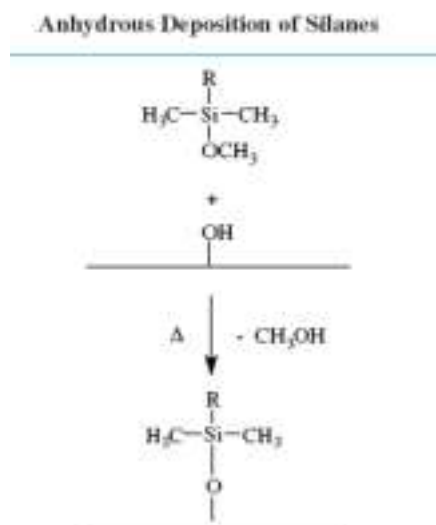
그림 8. 물 촉매 없는 메톡시 실란의 표면반응. 15
