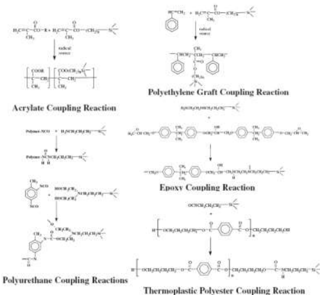
그림 15. 고분자와 기질표면과의 강한 결합을 위한 다양한 실란 반응들. 15
