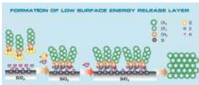
그림 6. 물의 존재하에서 축합반응을 통한 자기조립막 형성 과정. 9
