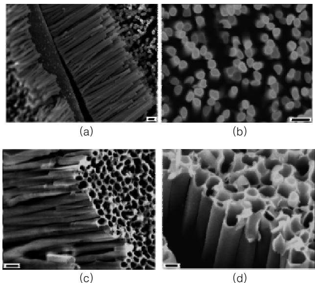
그림 11. 부분습윤에 의해 제조된 polystyrene( M_n = 30.5 kg/mol) 나노와이어 (a), (b)와 완전습윤에 의해 제조된 polystyrene 나노튜브 (c), (d). 74
