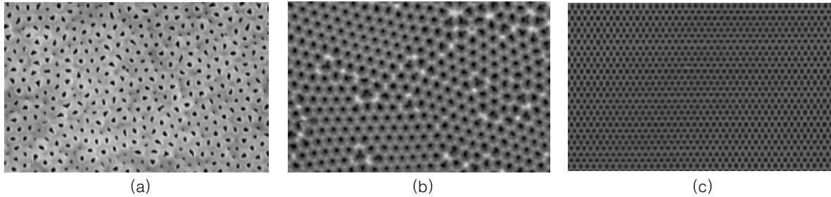
그림 7. 정렬되지 않은 다공성 알루미늄과 정렬된 다공성 알루미늄 비교. (a) 정렬되지 않은 다공성 알루미늄(disordered porous alumina), (b) 자기 정렬된 다공성 알루미늄(self-ordered porous alumina by 2-step anodization), (c) 임프린트 리소그래피에 의해 얻어진 완벽하게 정렬된 다공성 알루미늄(perfectly-ordered porous alumina by combination of imprint lithography and anodization).
