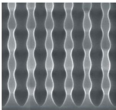
그림 4. 3D-마크로포러스 실리콘.
