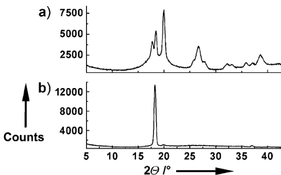
그림 23. PVDF 참조시료와 나노튜브의 X-ray 회절 결과: 나노튜브의 성장은 한쪽방향으로 결정성을 가지고 있음을 의미. 40
