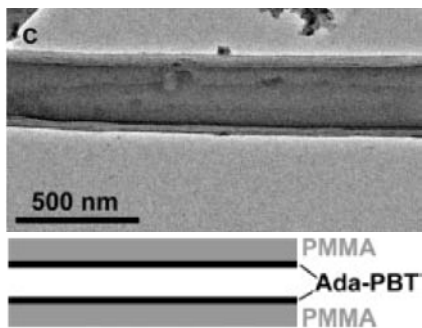
그림 19. 습윤법으로 제조된 PMMA/Ada-PBT의 2중층 막.
