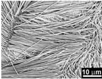
그림 12. 템플레이트-습윤법으로 제조된 PEEK 나노튜브.
