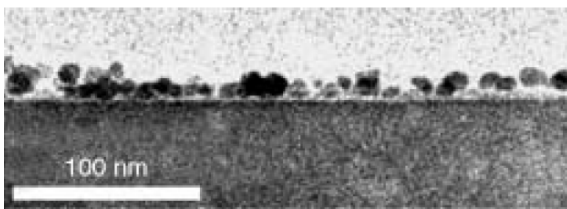
그림 24. 다공성 알루미늄에 습윤된 팔라듐/PLA 복합체의 극박막 단면 TEM 사진. 39
