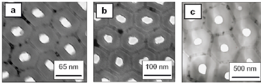
그림 6. 정렬된 다공성 알루미늄의 TEM image: (a) 황산조건, (b) 옥살산조건, (c) 인산조건.
