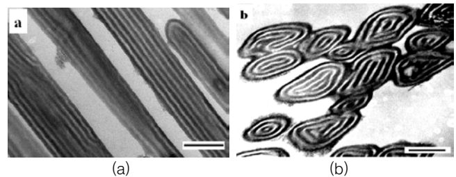
그림 21 다공성 알루미늄에서 성장한 PS- b -PBD lamellar 나노와이어의 TEM 사진. (a) 다공길이 방향 and (b) 다공 단면.
