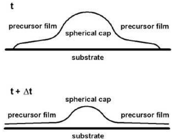
그림 8. 습윤에 의한 전구체막의 생성과정.
