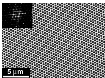
그림 3. 마크로포러스 실리콘.
