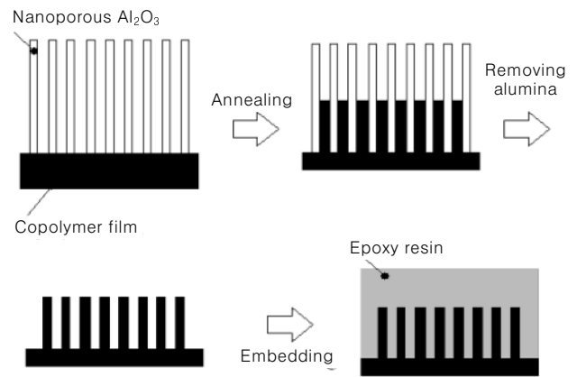
그림 20. PS- b -PBT 습윤법에 의한 제조공정.
