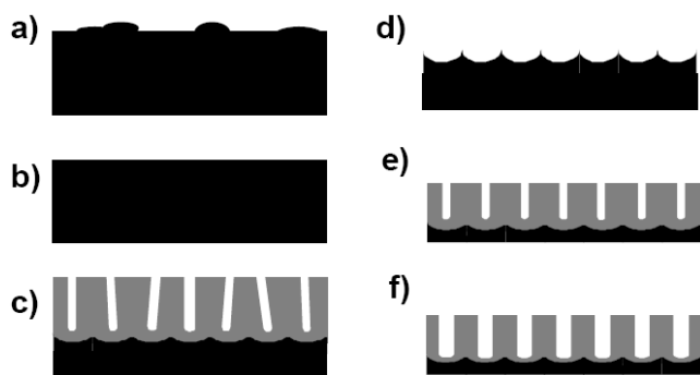
그림 5. 정렬된 다공성 알루미늄 제조법. (a) 알루미늄 금속시편, (b) 평탄한 표면을 얻기 위한 전기화학적 연마, (c) 1차 양극산화, (d) 양극산화된 알루미늄 제거, (e) 2차 양극산화, (f) 후처리 (다공의 크기제어).
