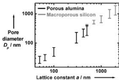
그림 1. 현재 이용가능한 다공성 알루미나와 마크로포러스 실리콘의 다공크기와 다공-다공거리. 38,52
