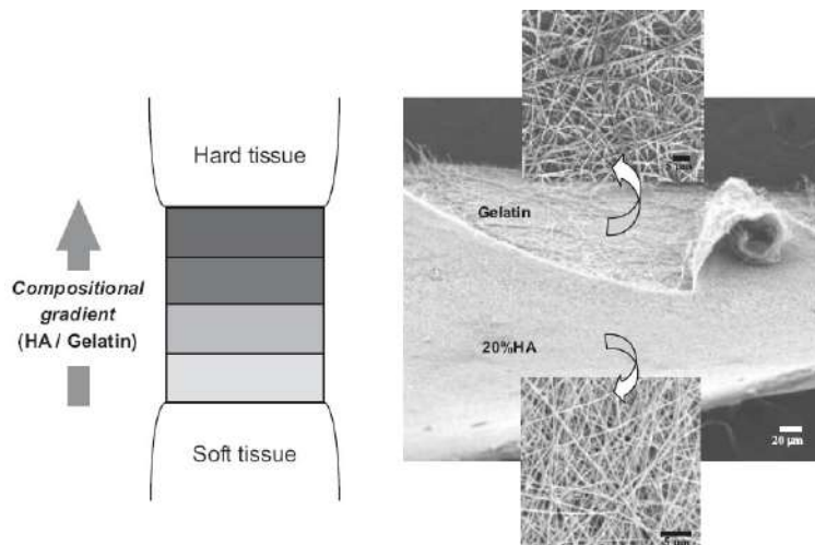
그림 7. (a) 생체모방법에 의한 젤라틴-아파타이트 나노하이브리드체를 전기나노방사장치를 이용하여 제조한 나노섬유의 투과전자현미경 사진(확대사진: HA나노결정립을 나타냄), (b) 적층구조로 제조된 나노섬유의 GBR멤브레인으로서의 응용. 26
