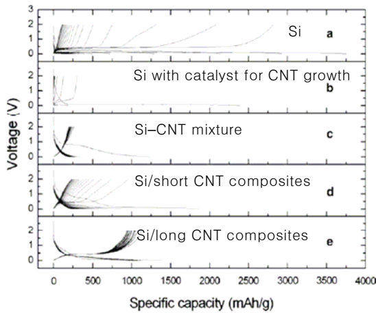
그림 6. 실리콘 입자위에 탄소나노튜브를 성장시킨 전극의 수명특성. 24
