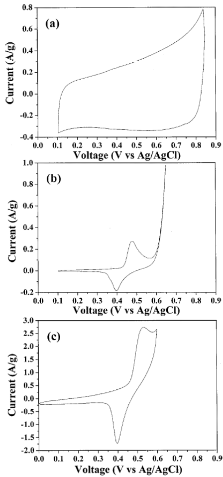
그림 8. 슈퍼커패시터 전극용 탄소나노튜브/전도성 고분자 복합체의 전기화학 특성 (a) 탄소나노튜브 (b) 폴리피롤 (c) 탄소나노튜브/폴리피롤 복합체. 29
