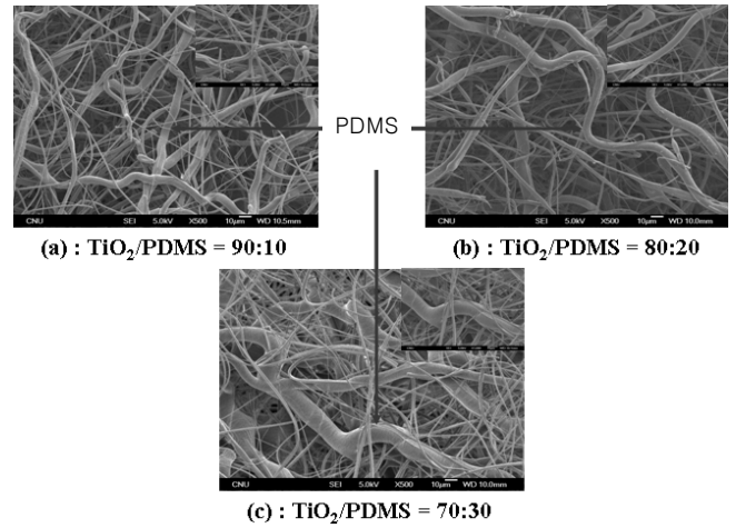
그림 12. SEM images of \text{TiO}_2 /PDMS composite fibers.
