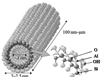
그림 1. Schematic representation of structure of imogolite nanofiber. 9
