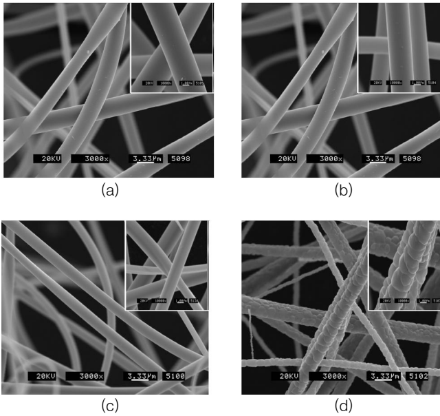
그림 10. SEM images of \text{TiO}_2 fibers : (a) Untreated, (b) 250 °C 3 h, (c) 600 °C 3 h, and (d) 1,300 °C 3 h.
